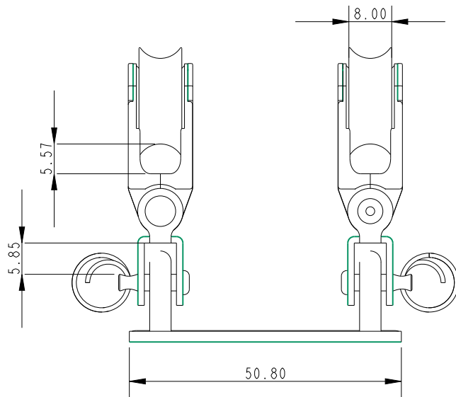
SCALE 1:1
